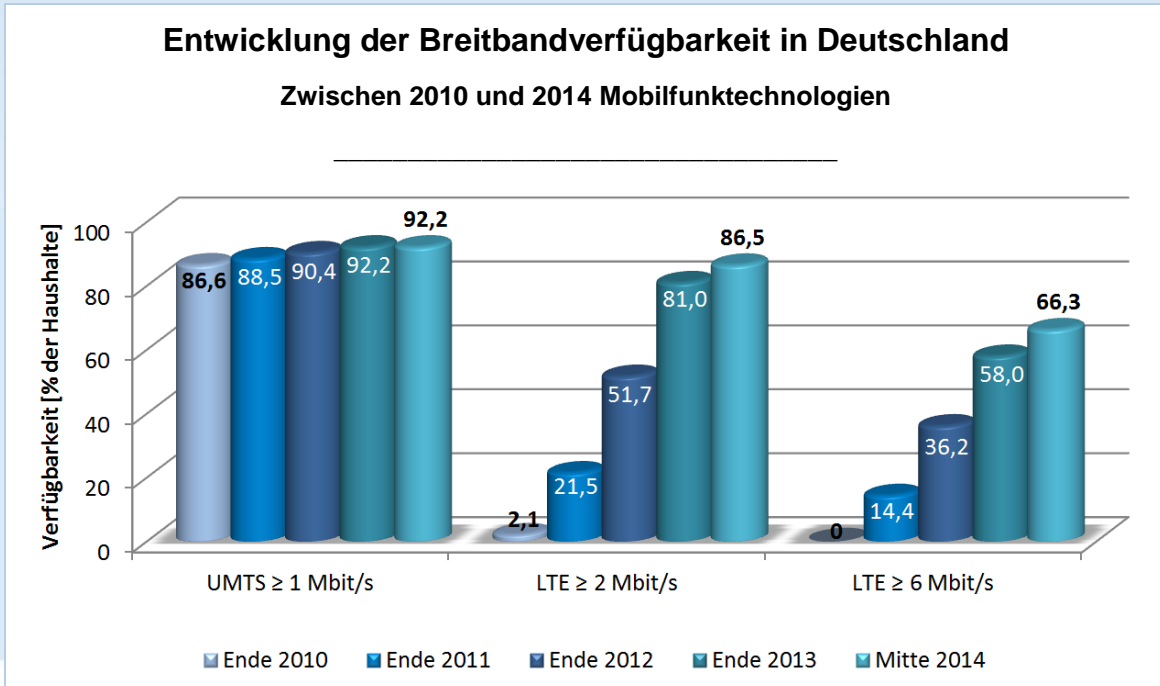
Abbildung 10: Entwicklung der Breitbandverfügbarkeit in Deutschland – Mobilfunktechnologien
